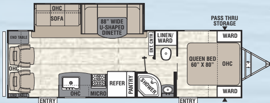
281 RLDSE / Exterior Length 31' 8"
