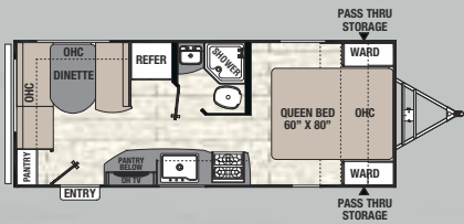
204 RD / Exterior Length 24' 7"
